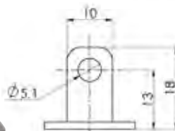
L字ステー寸法
