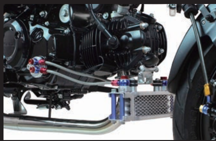
装着写真 (07-07-0423)
