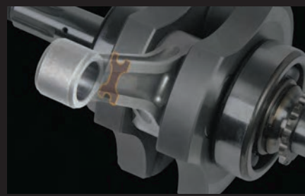
X断面形状コネクティングロッド採用
