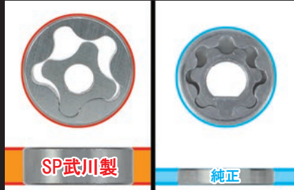
トロコイドローターの比較(左:SP武川製 右:純正)
