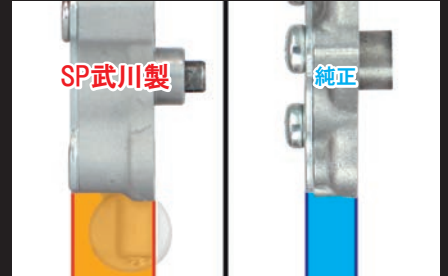
オイルポンプボディの厚み比較(左:SP武川製 右:純正)
