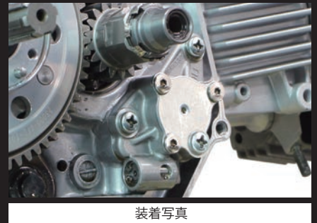
装着写真
