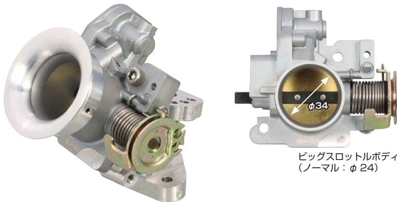
ノーマル(φ24)より口径を拡大した大型スロットルボディ。吸気量を大幅アップし、パワーアップに貢献します。
