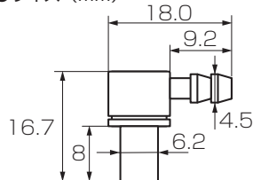
マニホールドのオイル / 負圧ニップルとして便利な L 型ニップルです。
