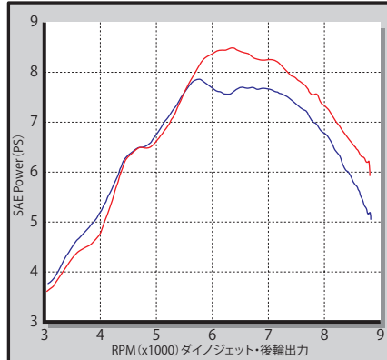
テスト車両:CT125(JA55) ■ノーマルピストン+N-15カムシャフト+ノーマルマフラー ■ノーマルピストン+ノーマルマフラー ダイノジェットによる後輪出力データは、実走行とは異なります。測定時の気温によっても大きく左右されます。参考データとしてご覧ください。
